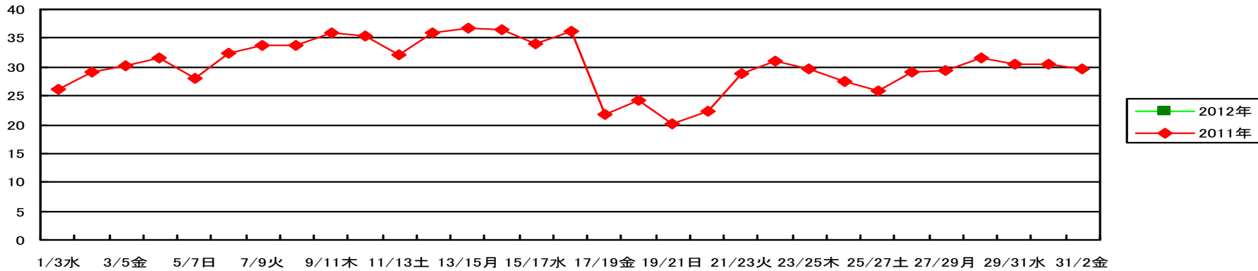
8月期 日最高気温 °C
