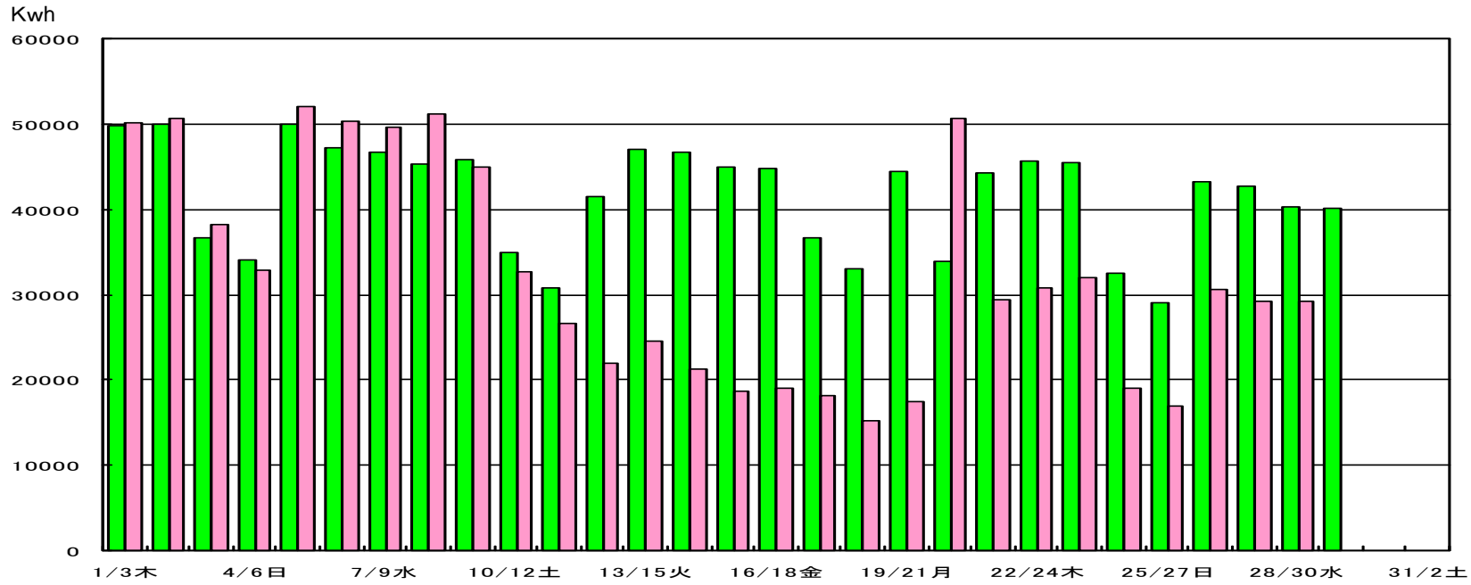
3月期 使用電力量推移 kWh
